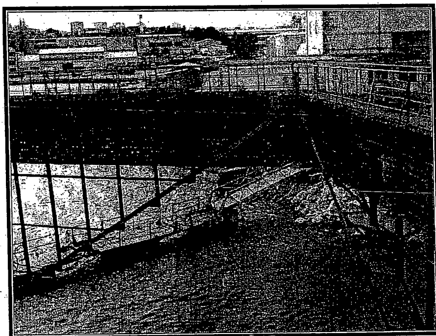
Slika 14. Korozijom oštećeni most
