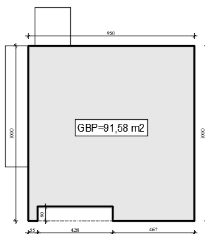
TLOCRT PRIZEMLJA
