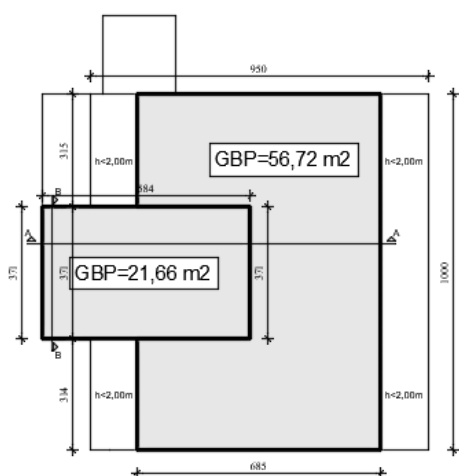
TLOCRT POTKROVLJA
