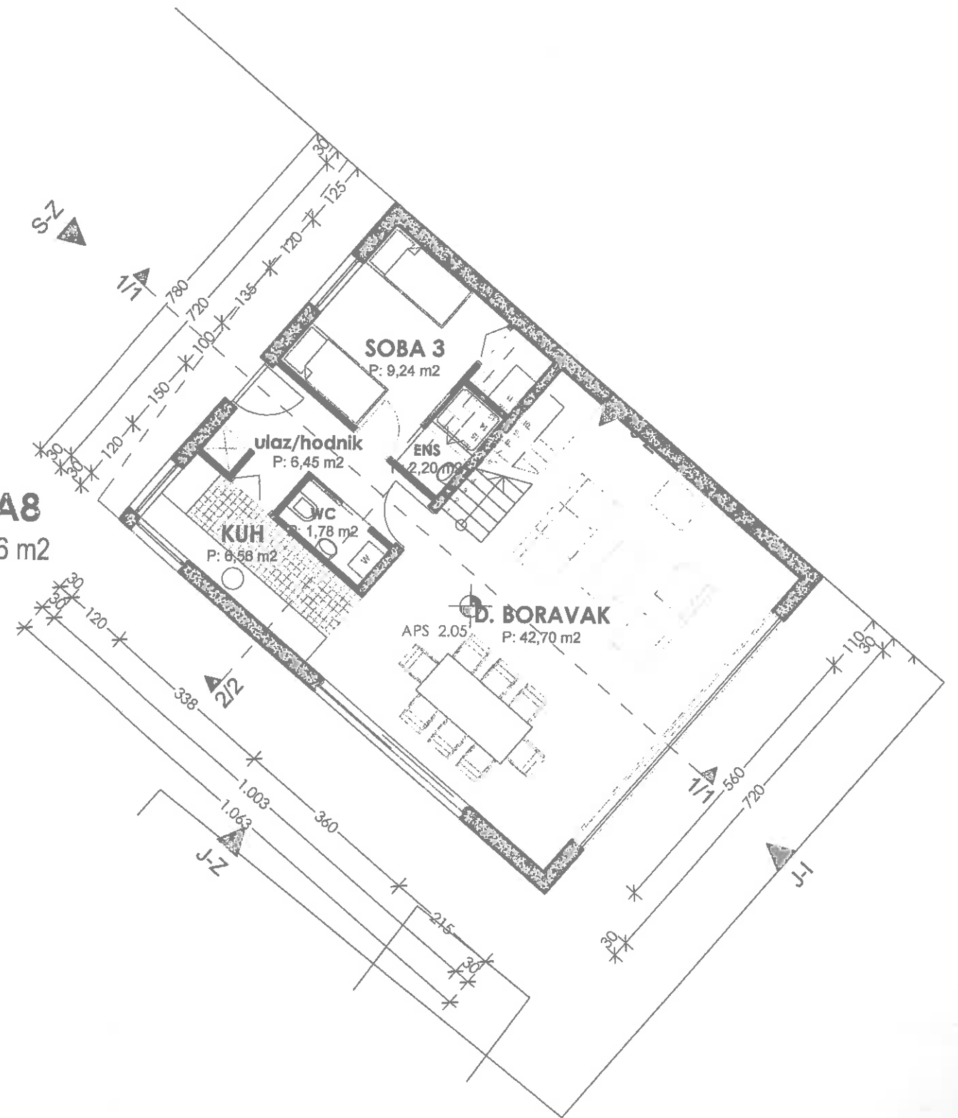
PRIZEMLJE - A8
