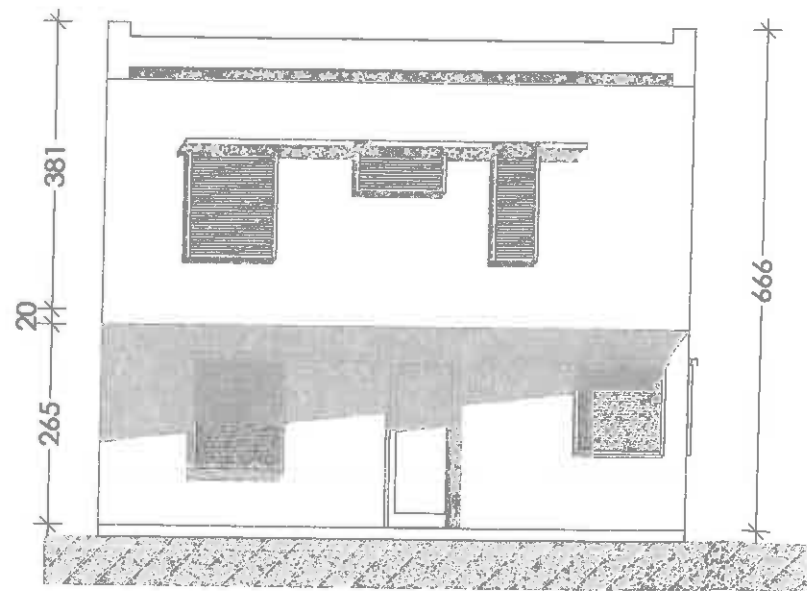
S-2 A8 1:100
