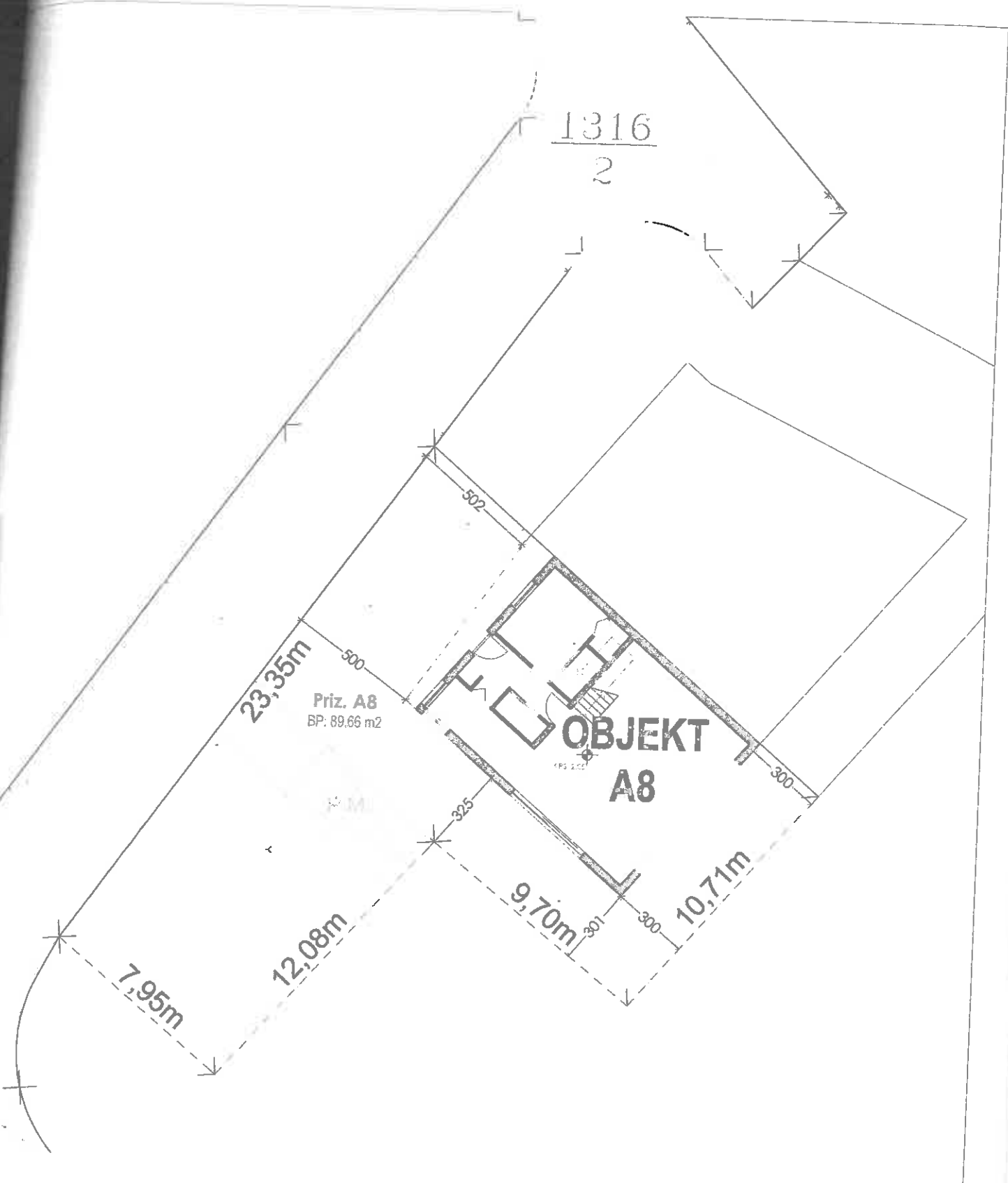
SITUACIJA - JEDINICA A8 1:200
