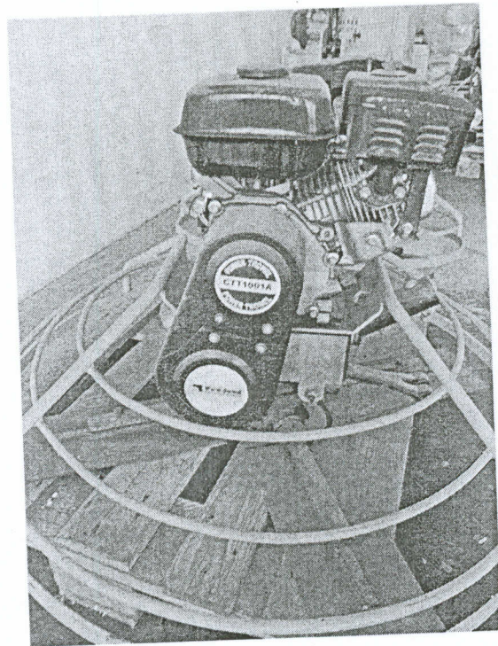
helikopter za beton vibro rbr 4
