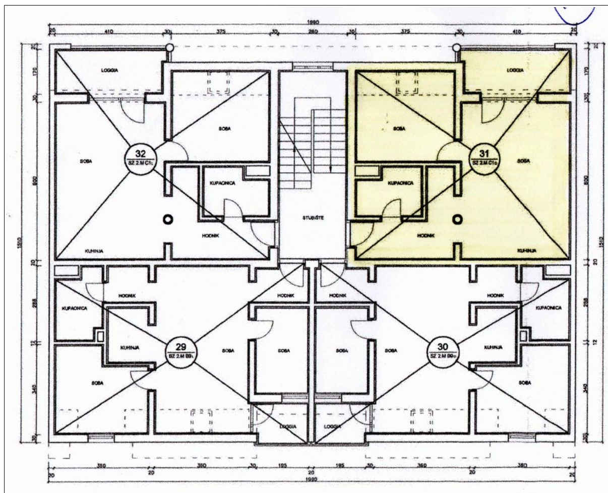
Tlocrt iz etažnog elaborata, predmetni stan označen žutom bojom
