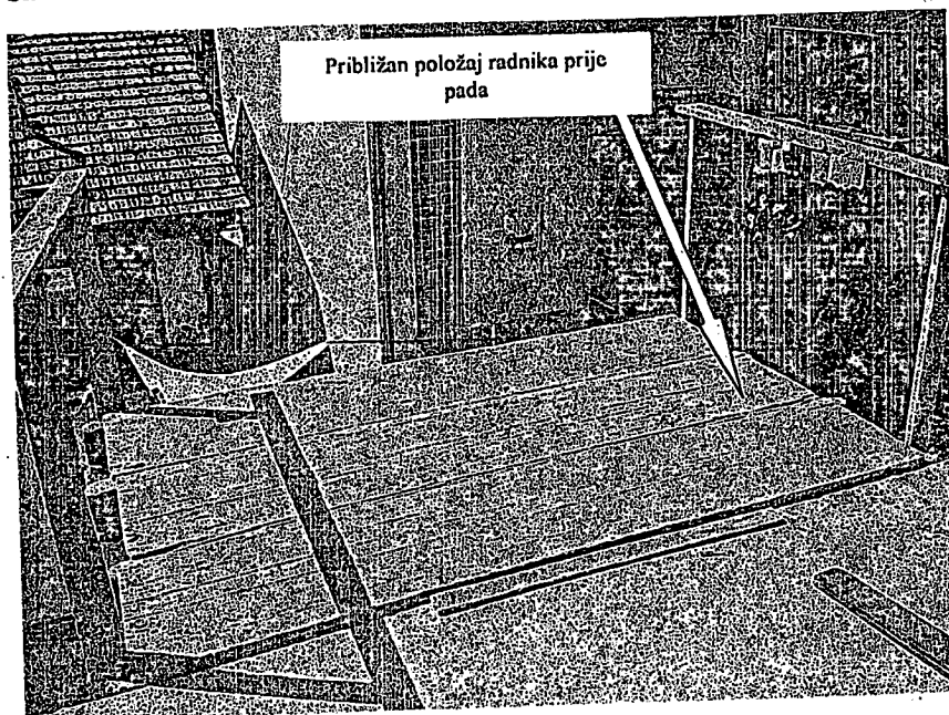
Slika 2 – Drveni konzolni istak (pogled iz prostorije)
