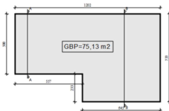
TLOCRT PRIZEMLJA
