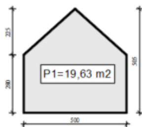
PRESJEK A-A
