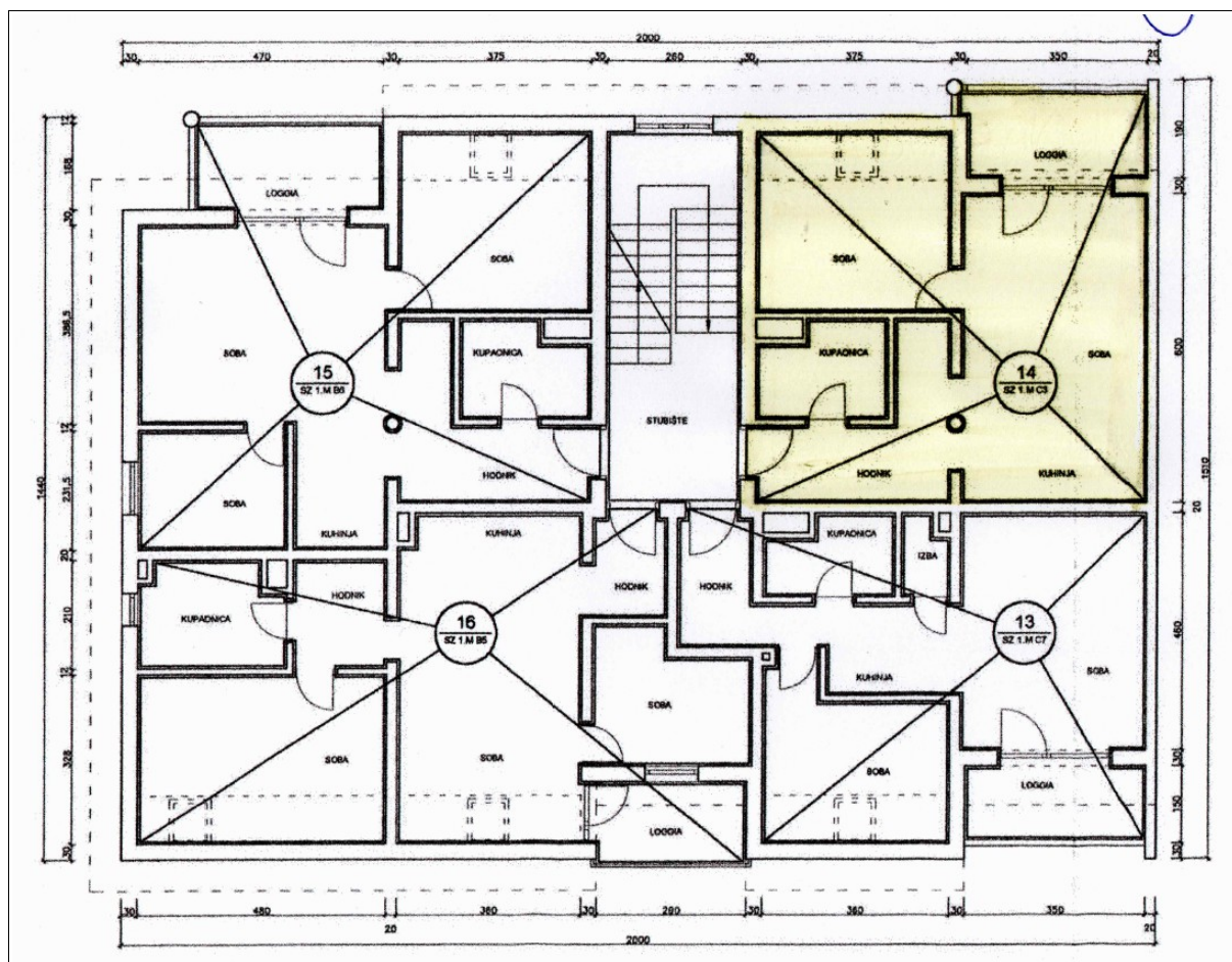
Tlocrt iz etažnog elaborata, predmetni stan označen žutom bojom
